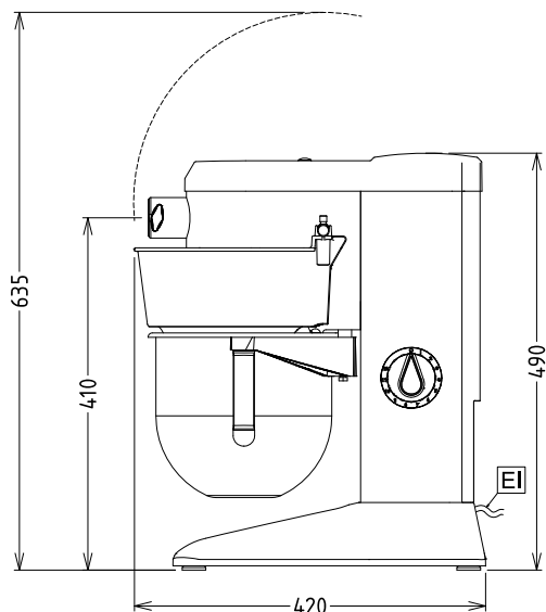
Zij aanzicht
